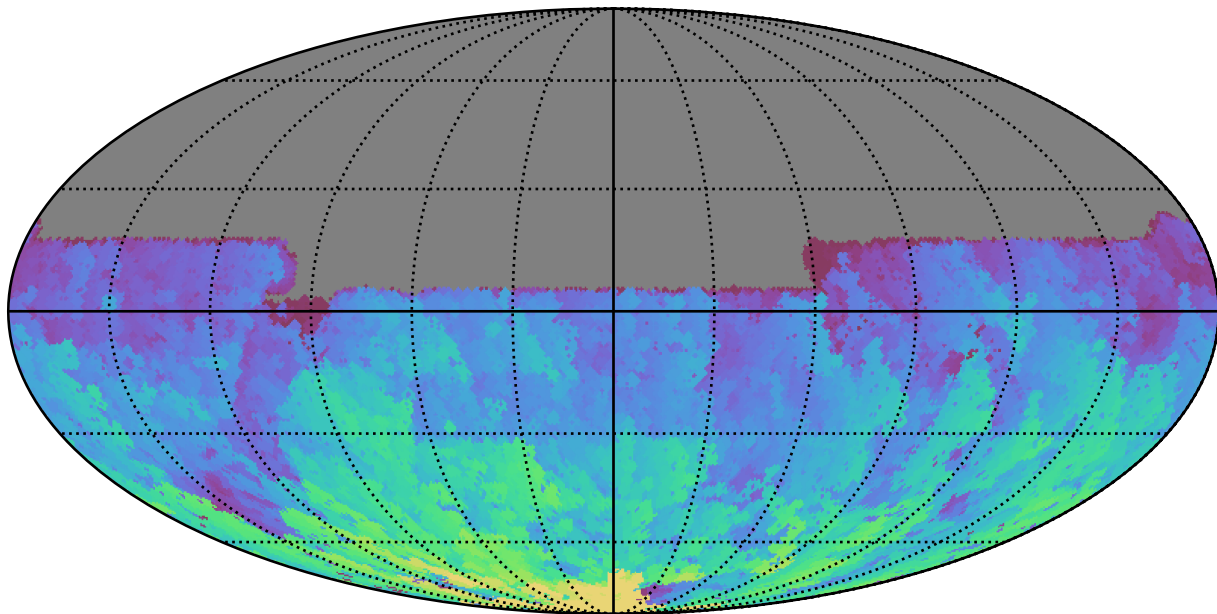
extra_ss_neo2_v3.4_10yrs All sky u band: Max HA
