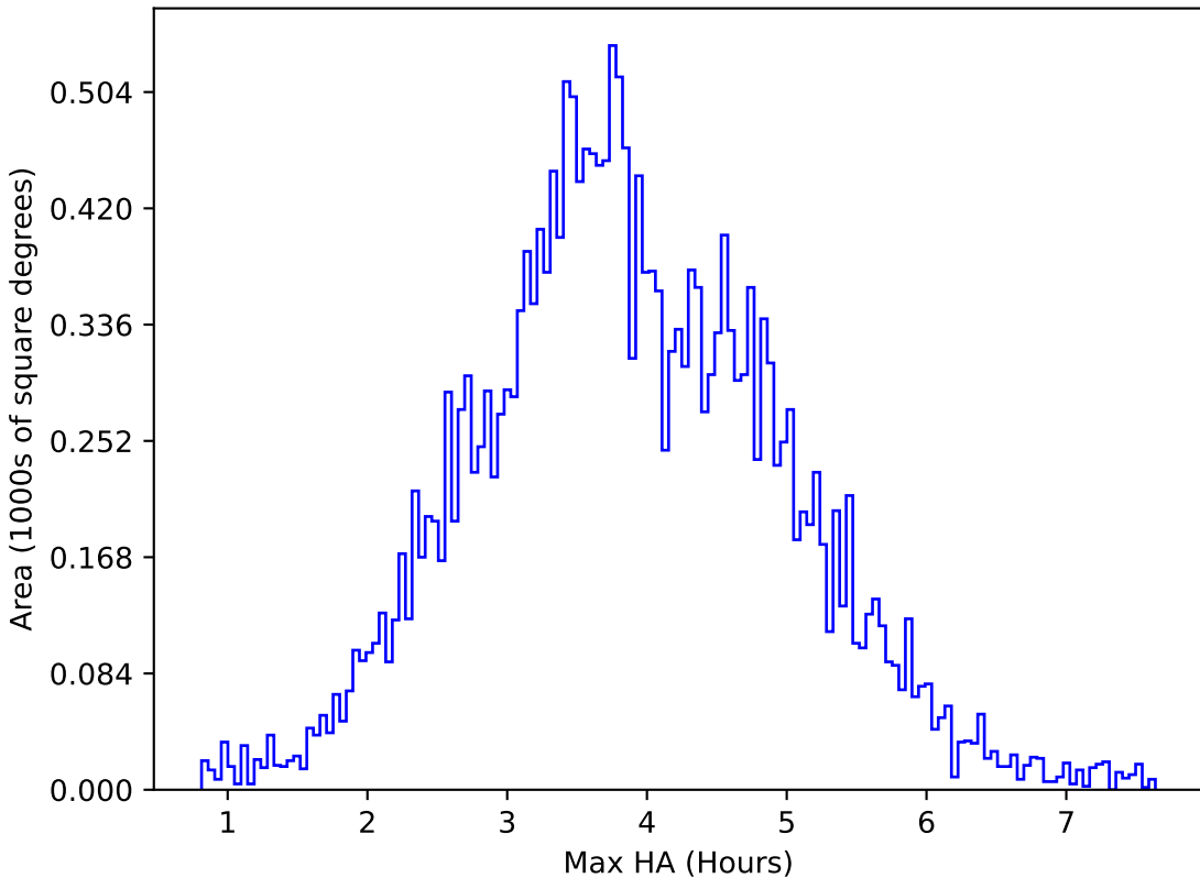
extra_ss_neo2_v3.4_10yrs All sky u band: Max HA
