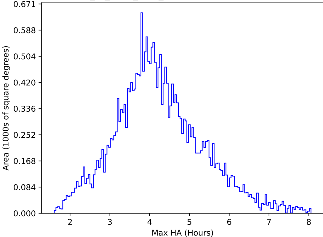
extra_ss_neo2_v3.4_10yrs All sky r band: Max HA
