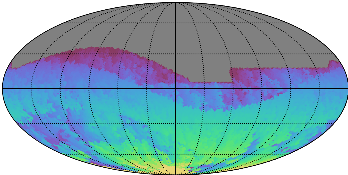
extra_ss_neo2_v3.4_10yrs All sky i band: Max HA
