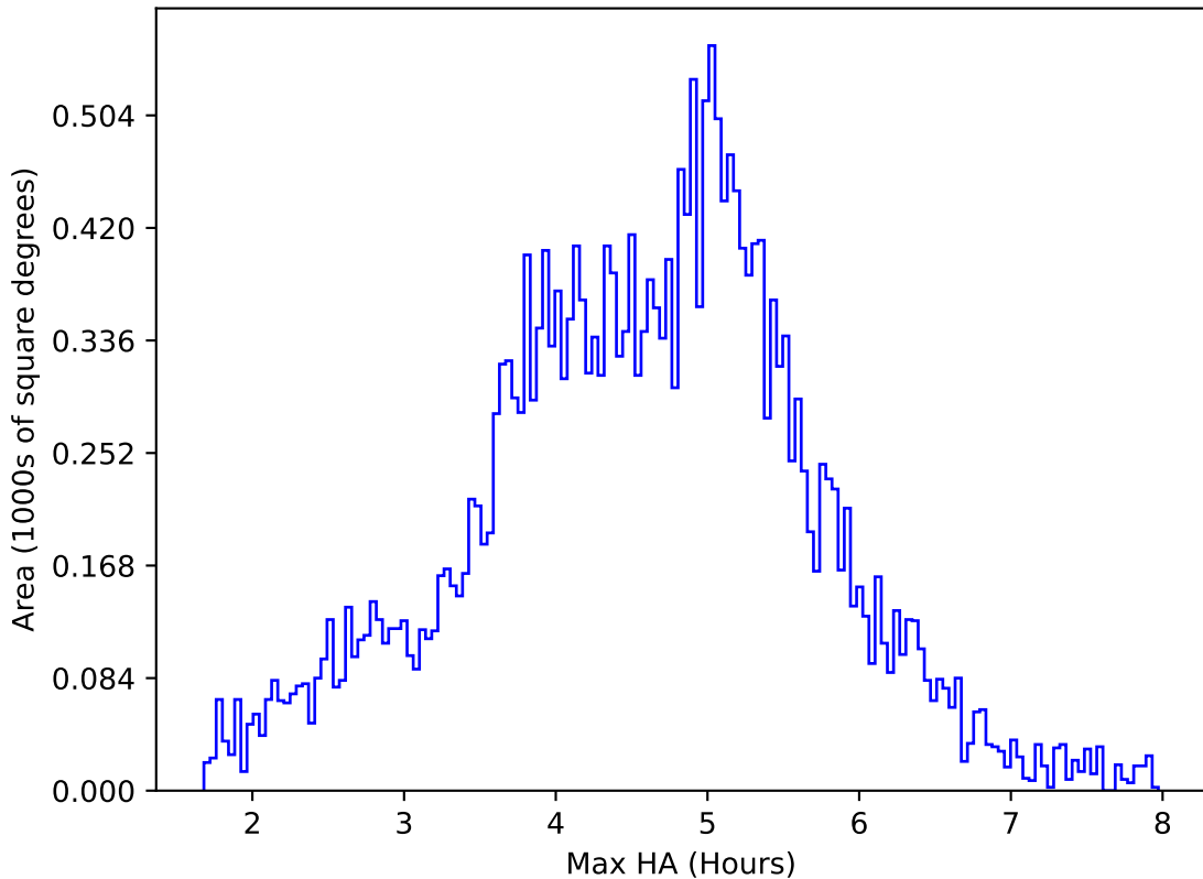
extra_ss_neo2_v3.4_10yrs All sky i band: Max HA
