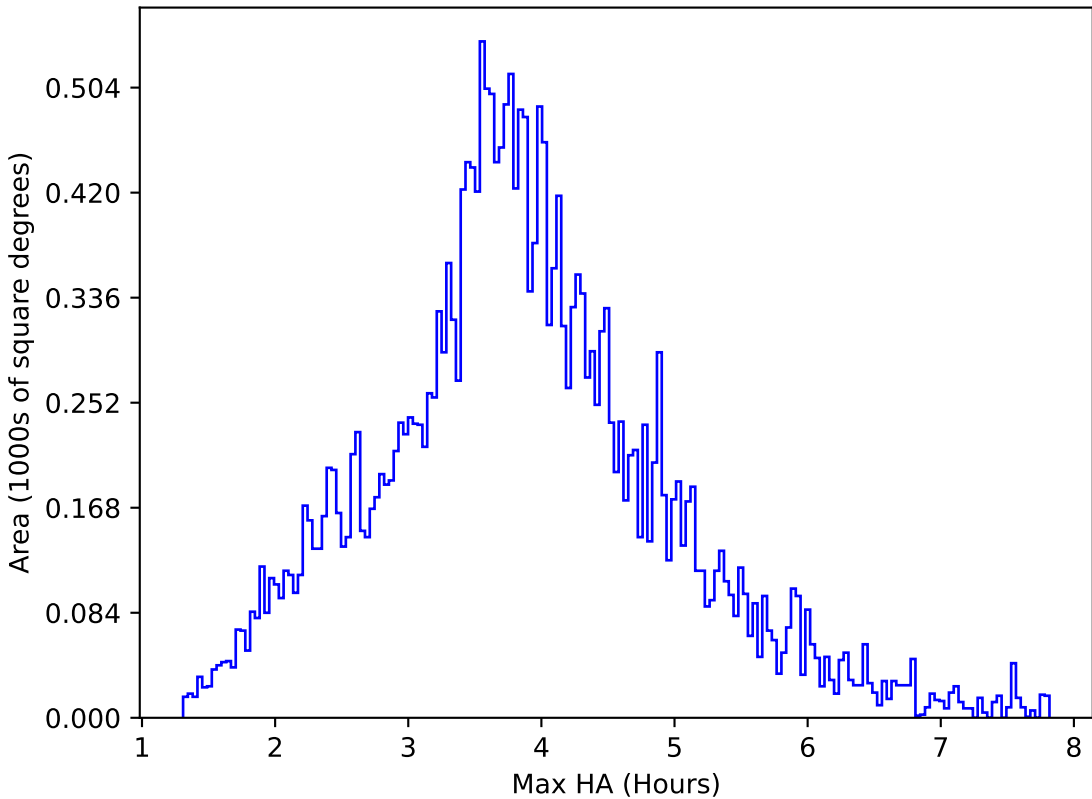
extra_ss_neo2_v3.4_10yrs All sky g band: Max HA
