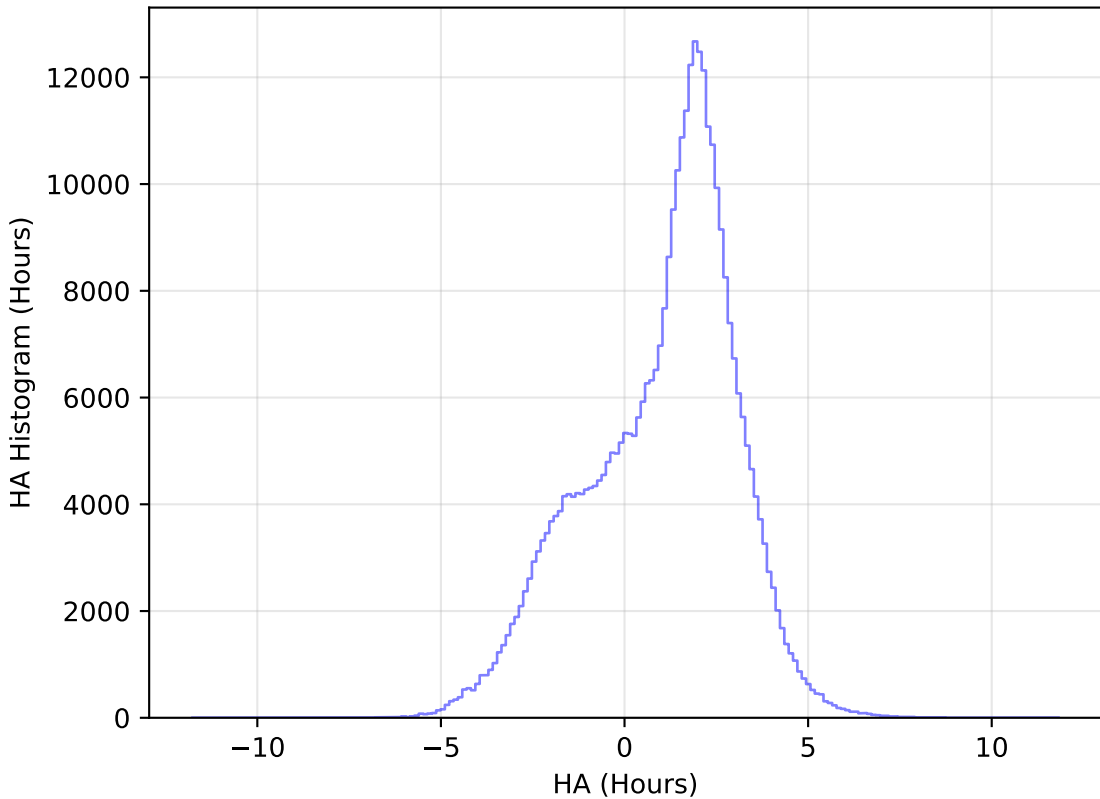
extra_ss_neo2_v3.4_10yrs WFD y band: HA Histogram
