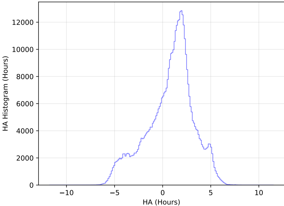
extra_ss_neo2_v3.4_10yrs All sky z band: HA Histogram
