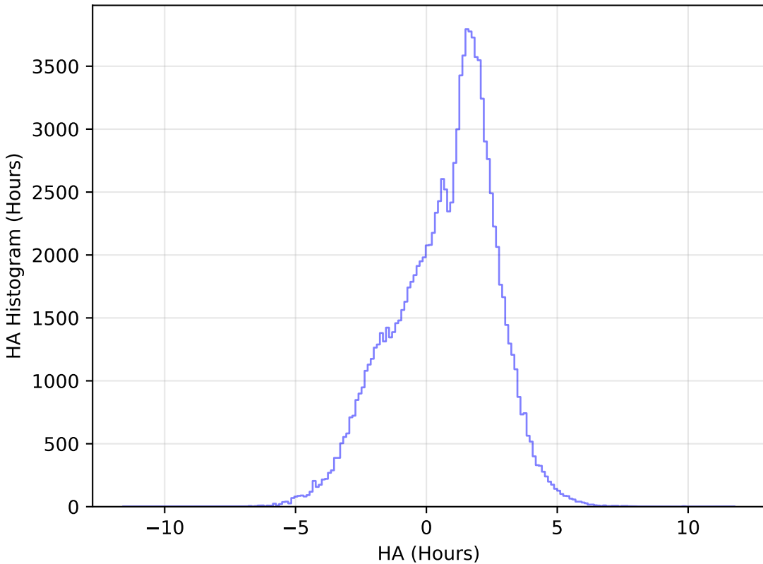
extra_ss_neo2_v3.4_10yrs All sky u band: HA Histogram
