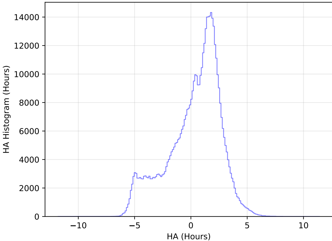
extra_ss_neo2_v3.4_10yrs All sky r band: HA Histogram
