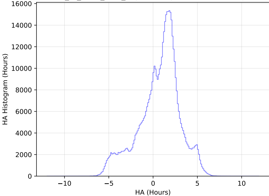
extra_ss_neo2_v3.4_10yrs All sky i band: HA Histogram
