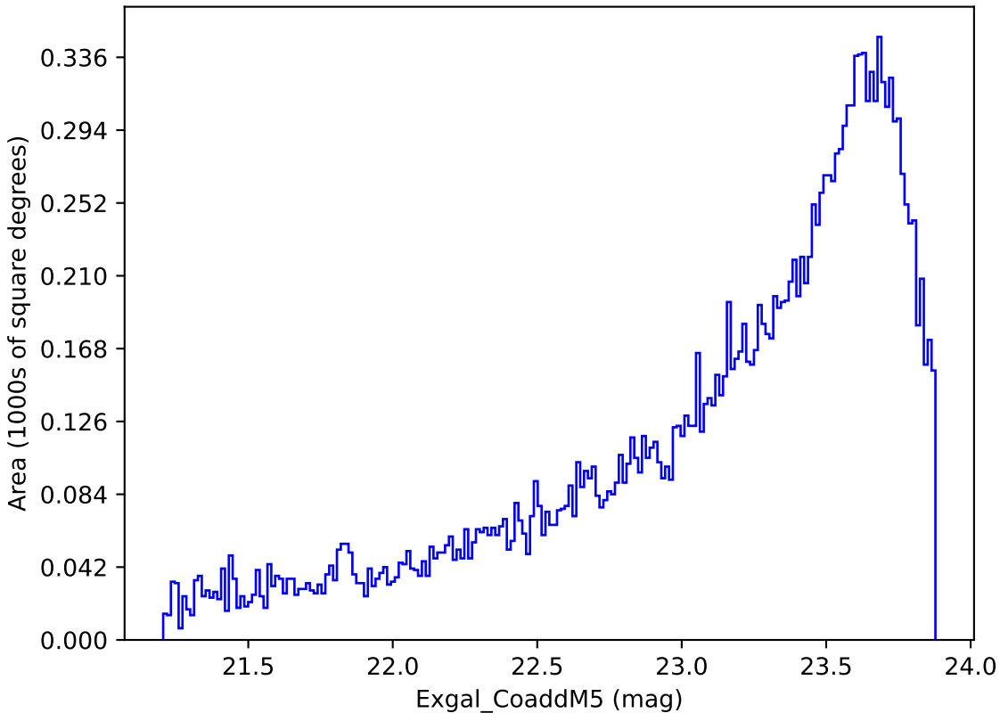
extra_ss_neo2_v3.4_10yrs Yr 3-4 y band: Exgal_CoaddM5
