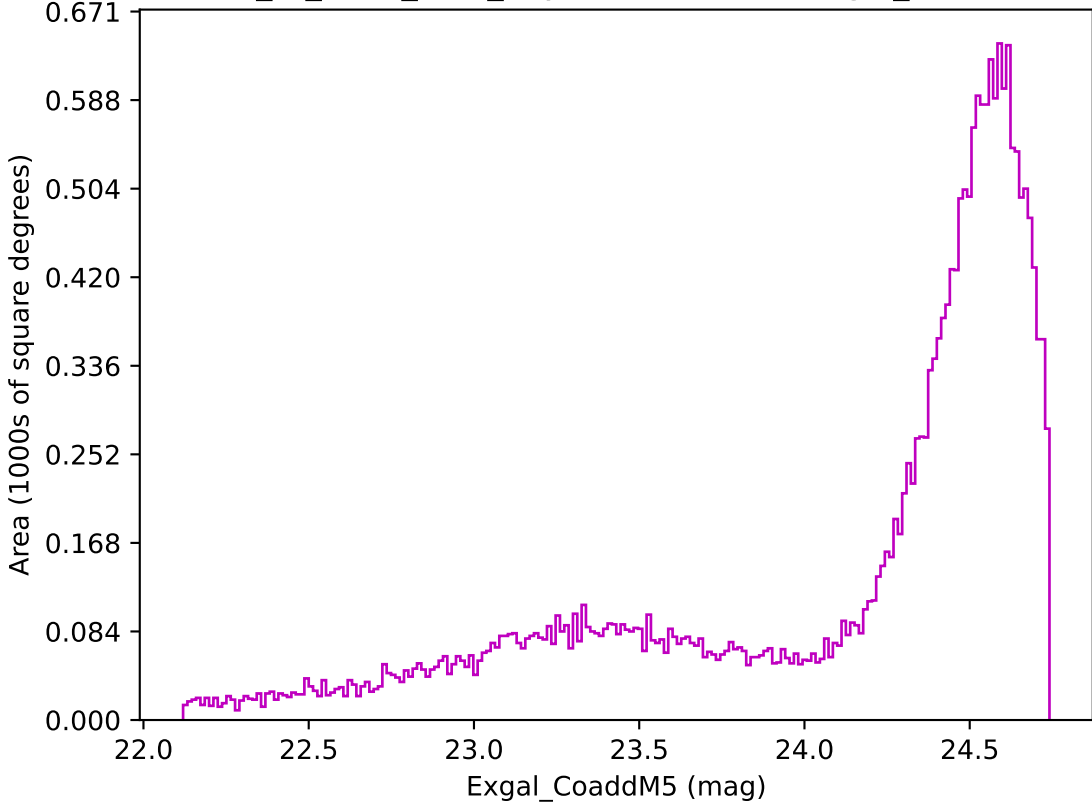
extra_ss_neo2_v3.4_10yrs Yr 1 z band: Exgal_CoaddM5
