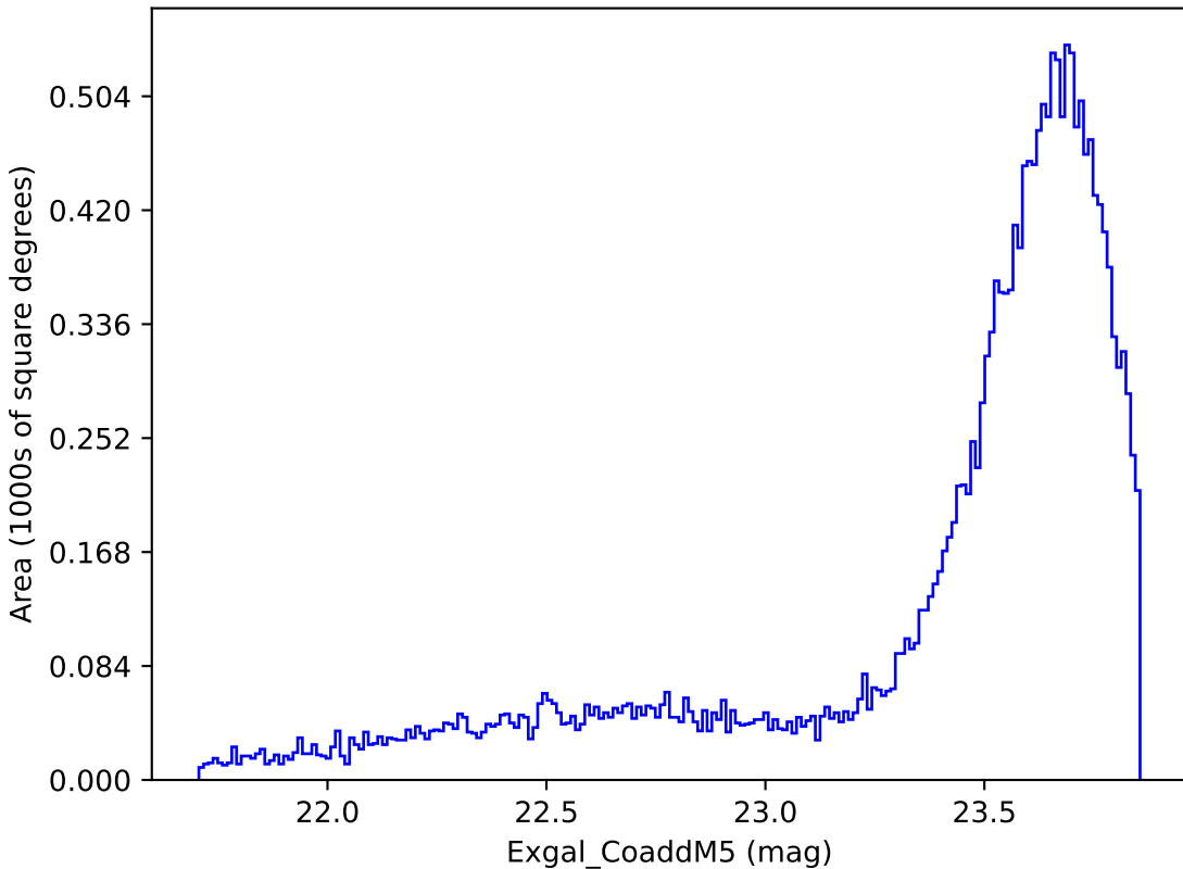
extra_ss_neo2_v3.4_10yrs Yr 1 y band: Exgal_CoaddM5
