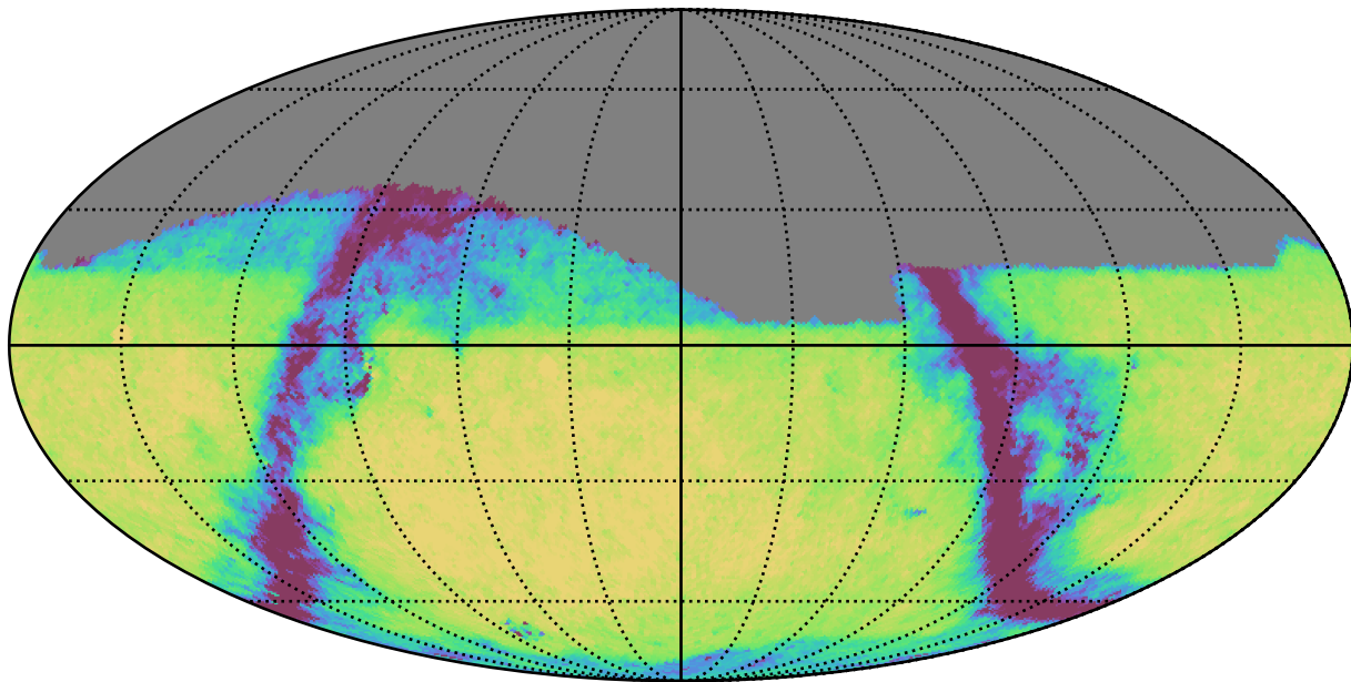
extra_ss_neo2_v3.4_10yrs Yr 1 r band: Exgal_CoaddM5
