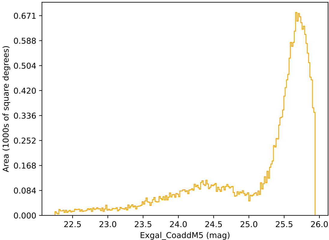
extra_ss_neo2_v3.4_10yrs Yr 1 r band: Exgal_CoaddM5
