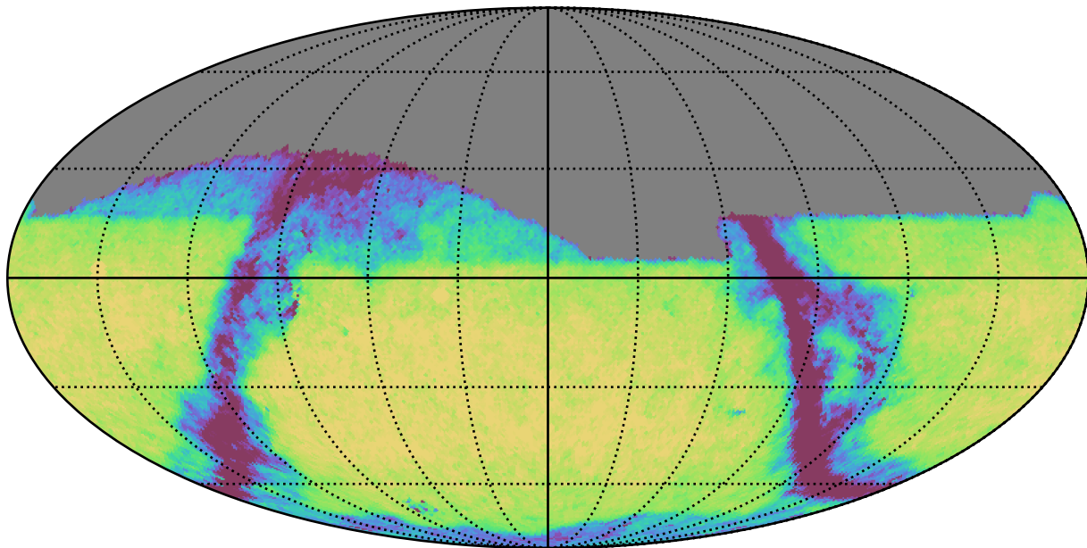
extra_ss_neo2_v3.4_10yrs Yr 1 i band: Exgal_CoaddM5
