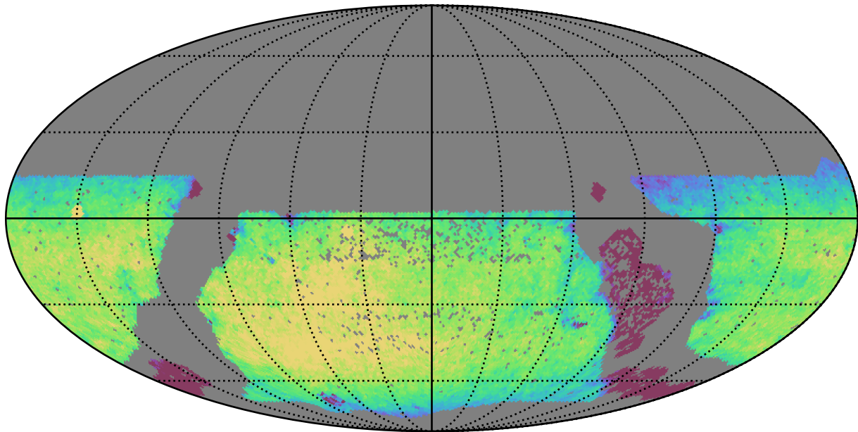
extra_ss_neo2_v3.4_10yrs WFD y band: Exgal_CoaddM5
