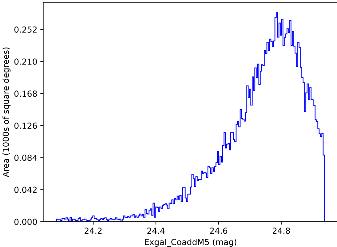
extra_ss_neo2_v3.4_10yrs WFD y band: Exgal_CoaddM5
