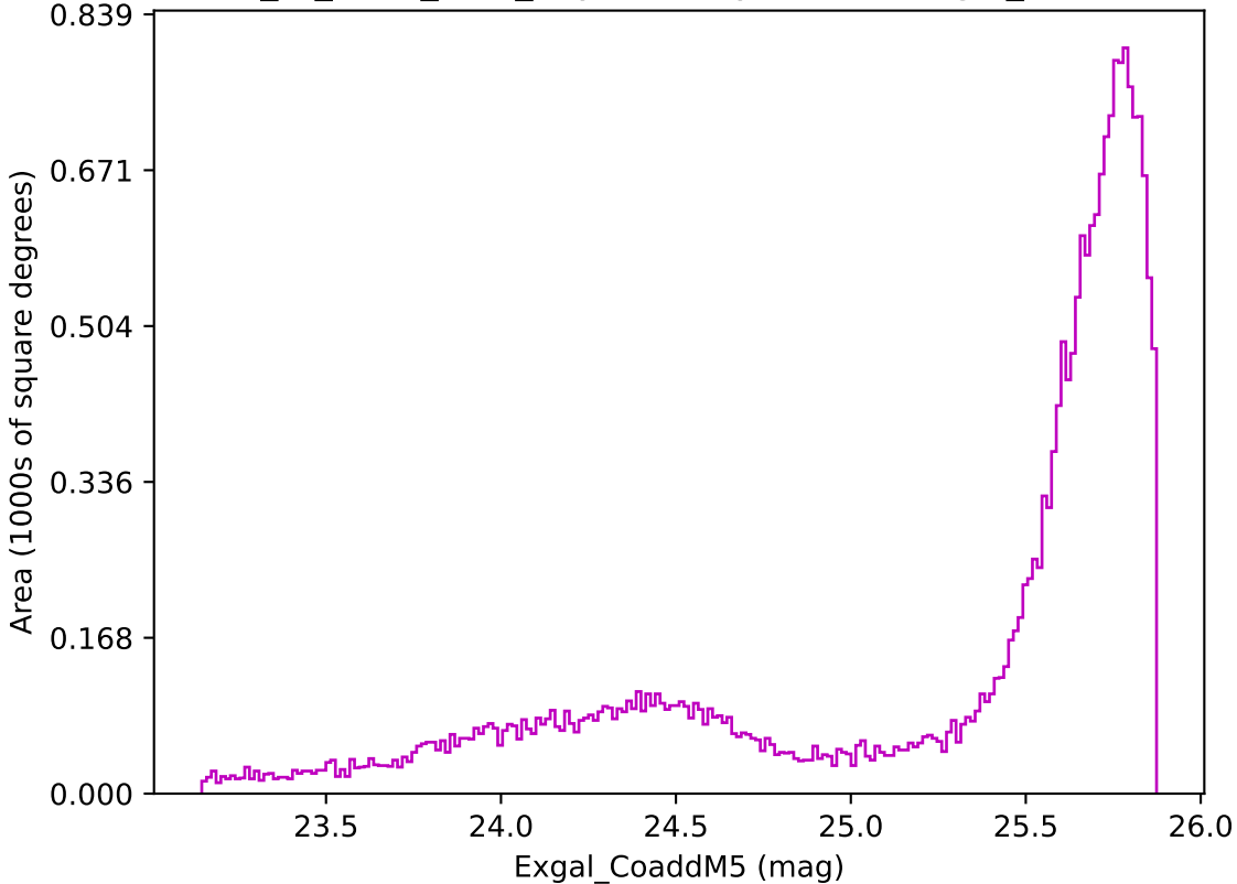
extra_ss_neo2_v3.4_10yrs All sky z band: Exgal_CoaddM5
