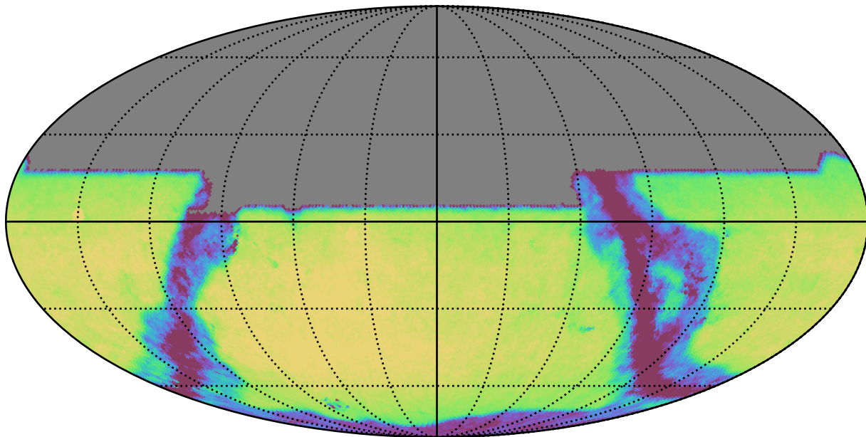
extra_ss_neo2_v3.4_10yrs All sky y band: Exgal_CoaddM5
