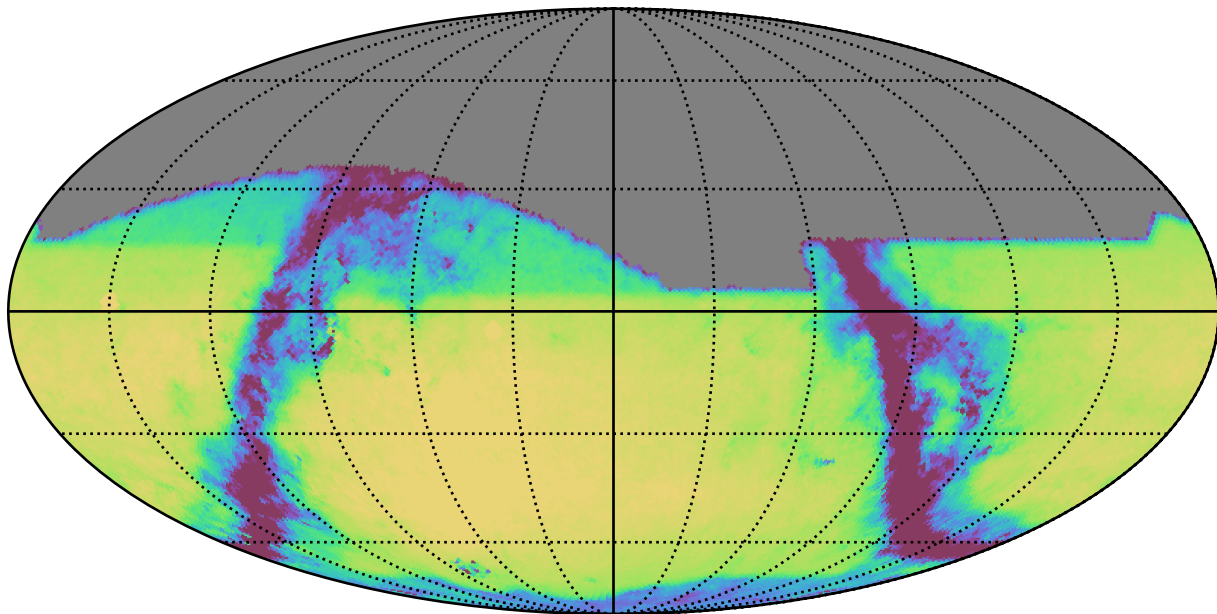
extra_ss_neo2_v3.4_10yrs All sky r band: Exgal_CoaddM5
