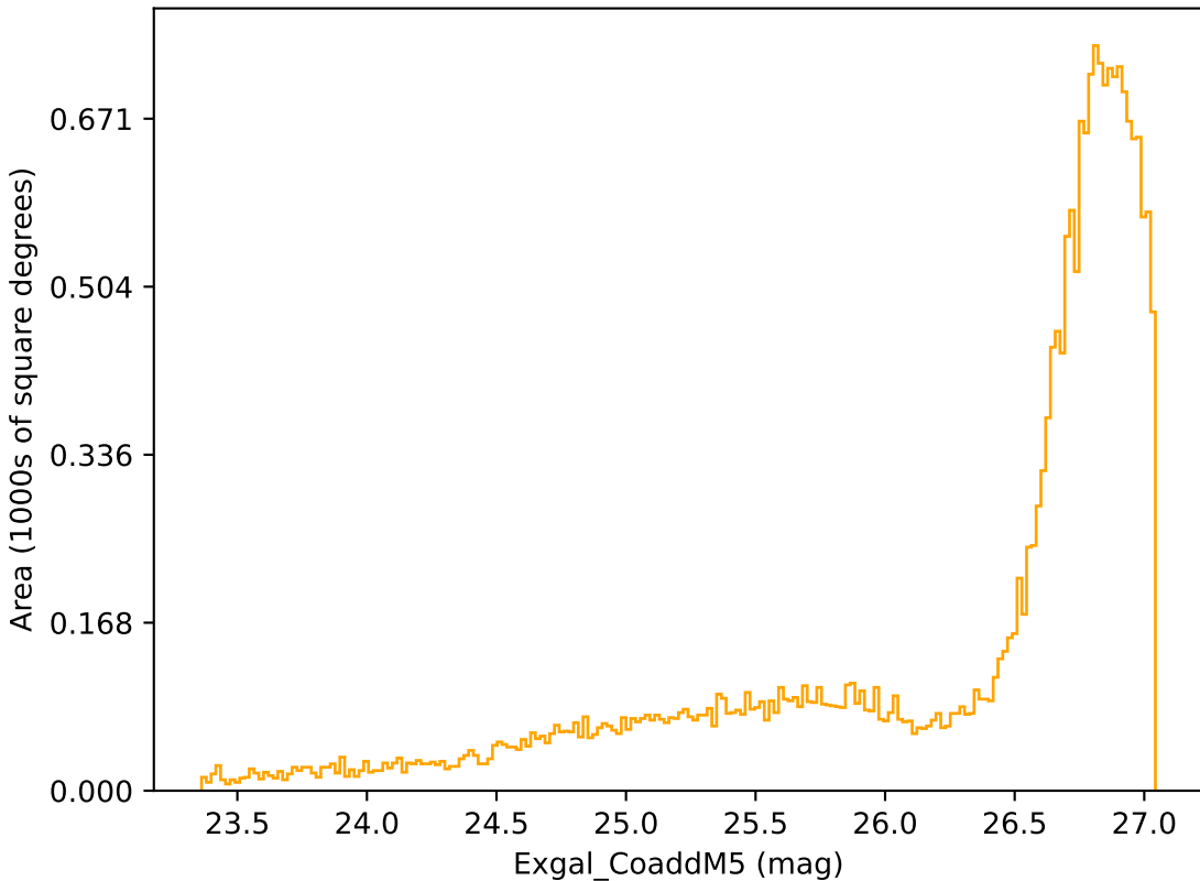
extra_ss_neo2_v3.4_10yrs All sky r band: Exgal_CoaddM5
