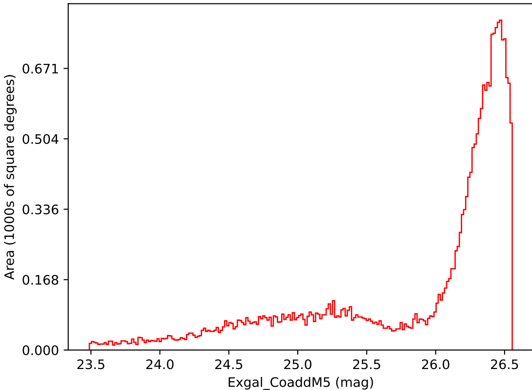
extra_ss_neo2_v3.4_10yrs All sky i band: Exgal_CoaddM5
