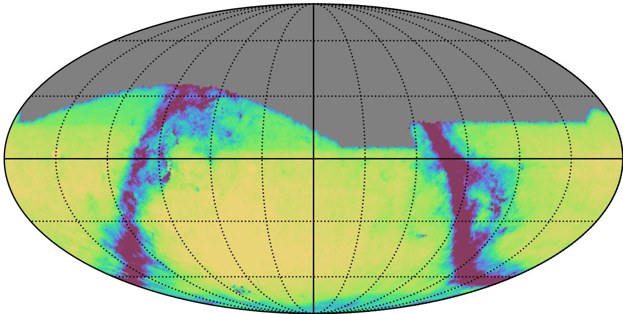
extra_ss_neo2_v3.4_10yrs All sky g band: Exgal_CoaddM5
