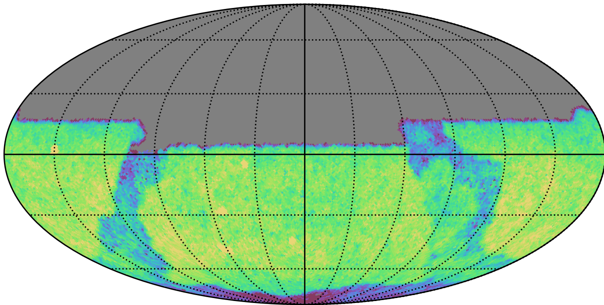
extra_ss_neo2_v3.4_10yrs Yr 1 y band: CoaddM5
