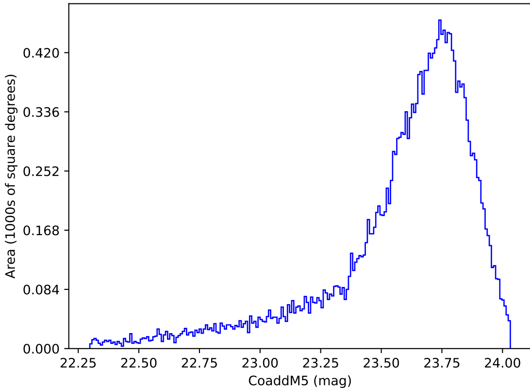
extra_ss_neo2_v3.4_10yrs Yr 1 y band: CoaddM5
