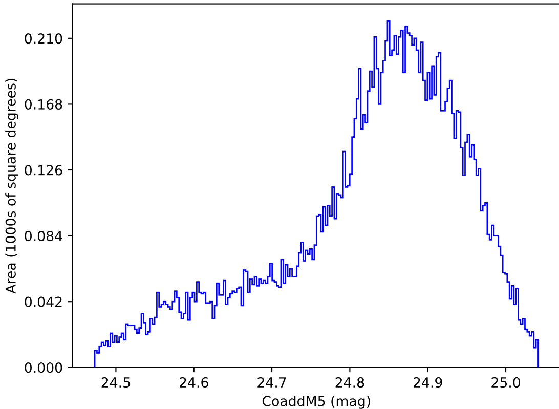
extra_ss_neo2_v3.4_10yrs WFD y band: CoaddM5
