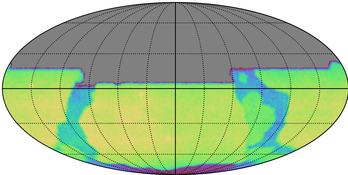
extra_ss_neo2_v3.4_10yrs All sky y band: CoaddM5
