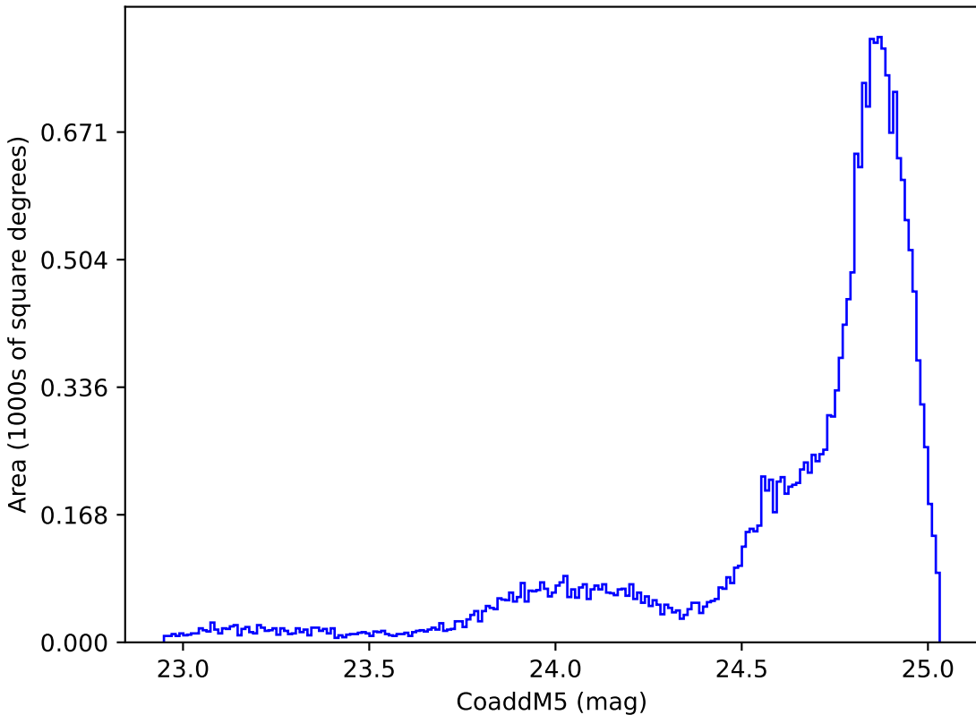
extra_ss_neo2_v3.4_10yrs All sky y band: CoaddM5
