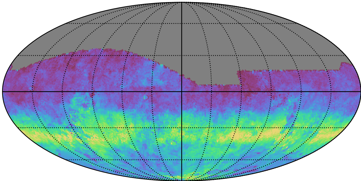
extra_ss_neo2_v3.4_10yrs All sky g band: AngleRms rotSkyPos
