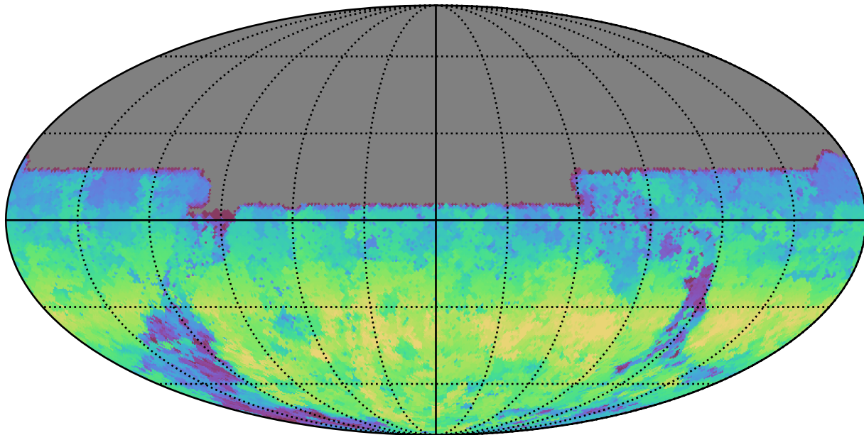
extra_ss_neo2_v3.4_10yrs All sky u band: AngleRange rotSkyPos
