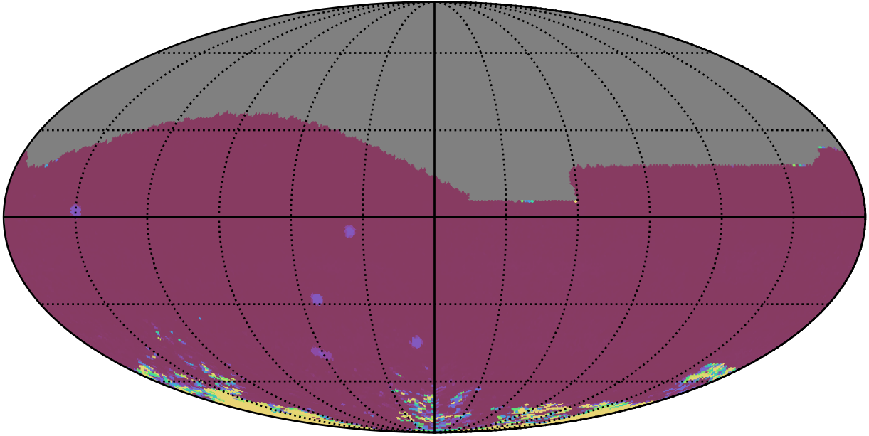
extra_ss_neo2_v3.4_10yrs All sky iz bands: 75th Percentile Intranight Timespan
