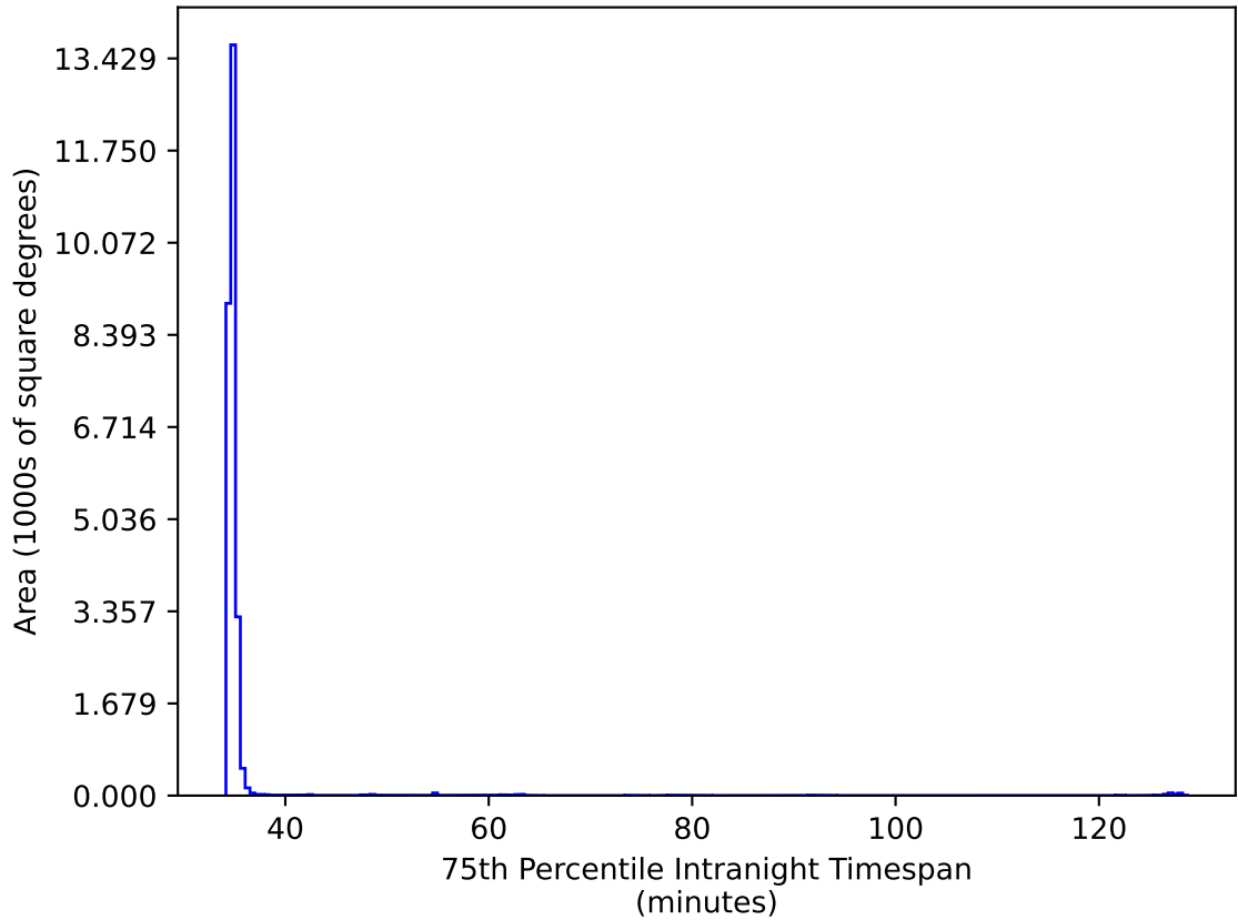
extra_ss_neo2_v3.4_10yrs All sky iz bands: 75th Percentile Intranight Timespan
