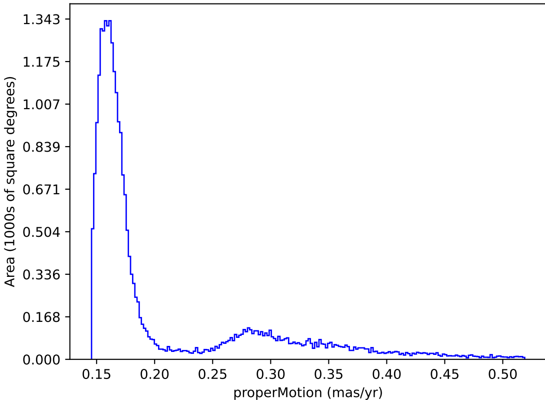
extra_ss_neo2_v3.4_10yrs : properMotion
