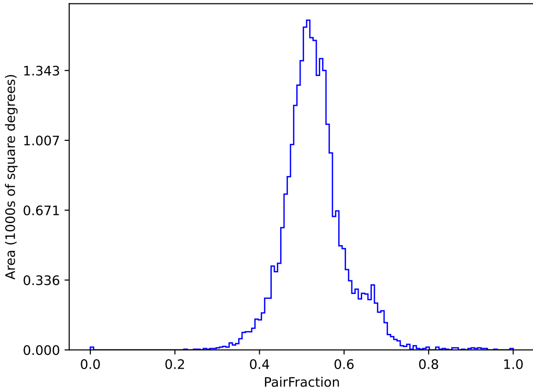
extra_ss_neo2_v3.4_10yrs (g or r or i): PairFraction
