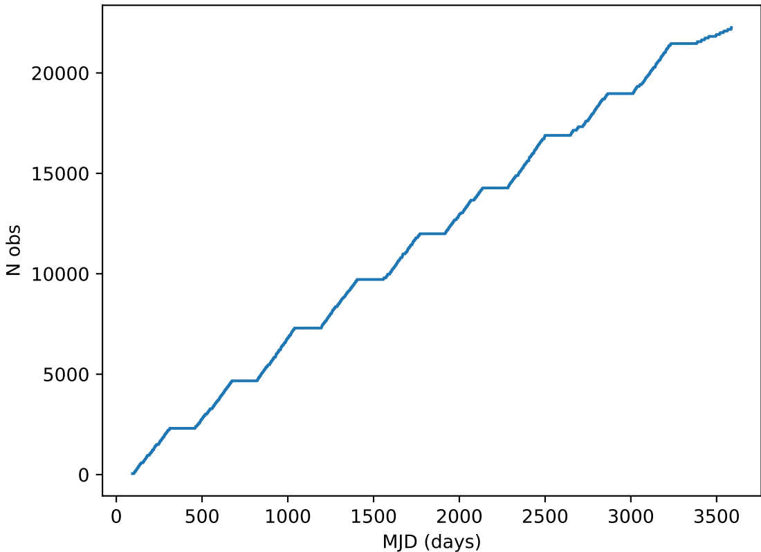
extra_ss_neo2_v3.4_10yrs note like DD:ECDFS%: Cumulative
