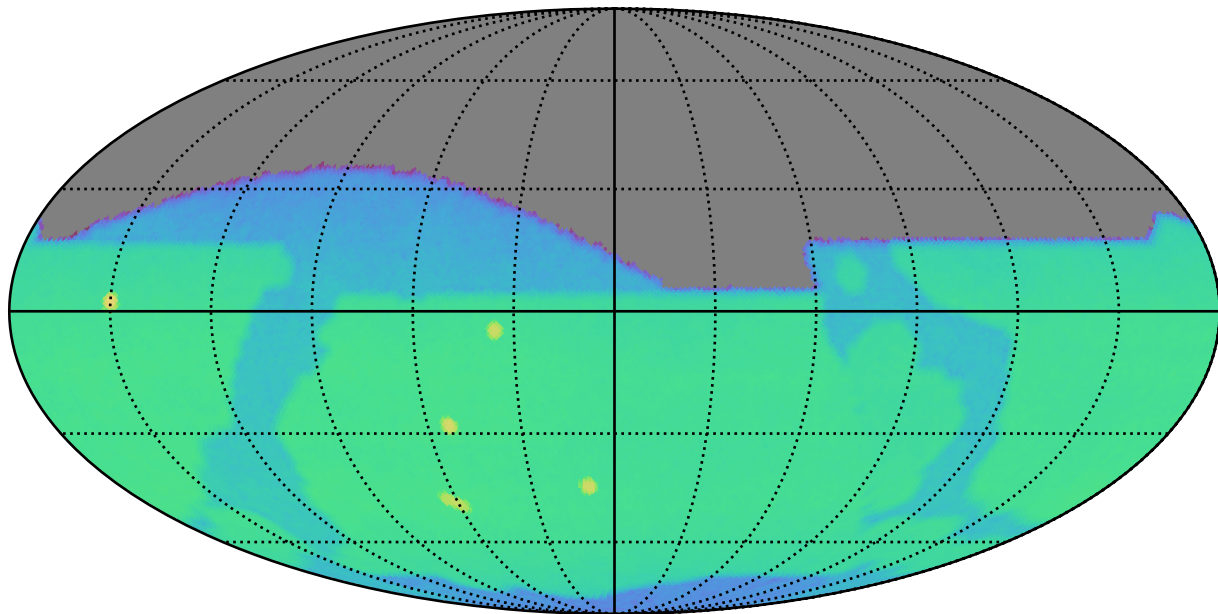
extra_ss_neo2_v3.4_10yrs z: CoaddM5
