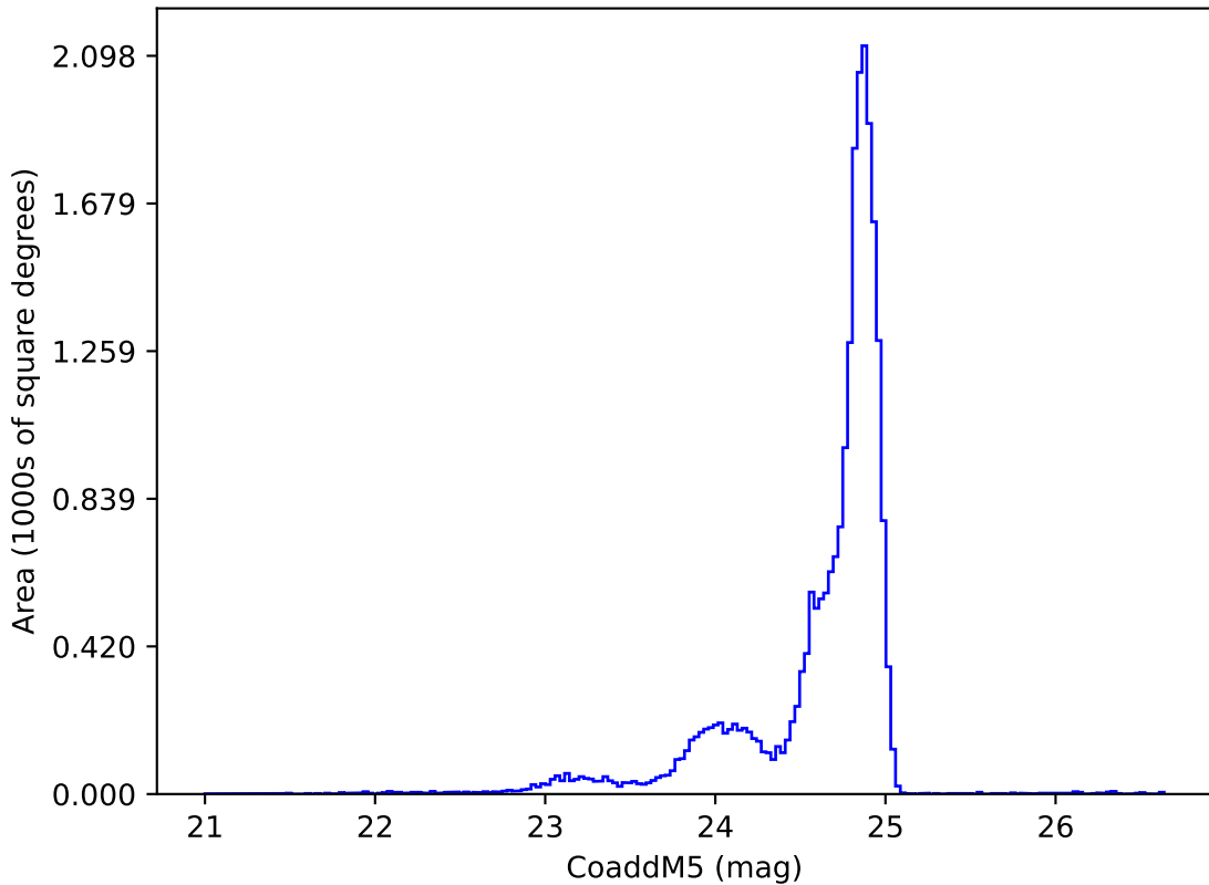
extra_ss_neo2_v3.4_10yrs y: CoaddM5
