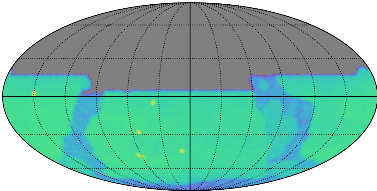
extra_ss_neo2_v3.4_10yrs u: CoaddM5
