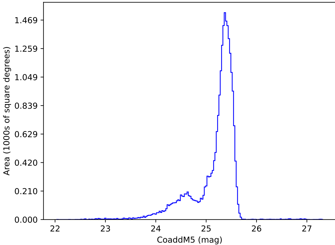
extra_ss_neo2_v3.4_10yrs u: CoaddM5
