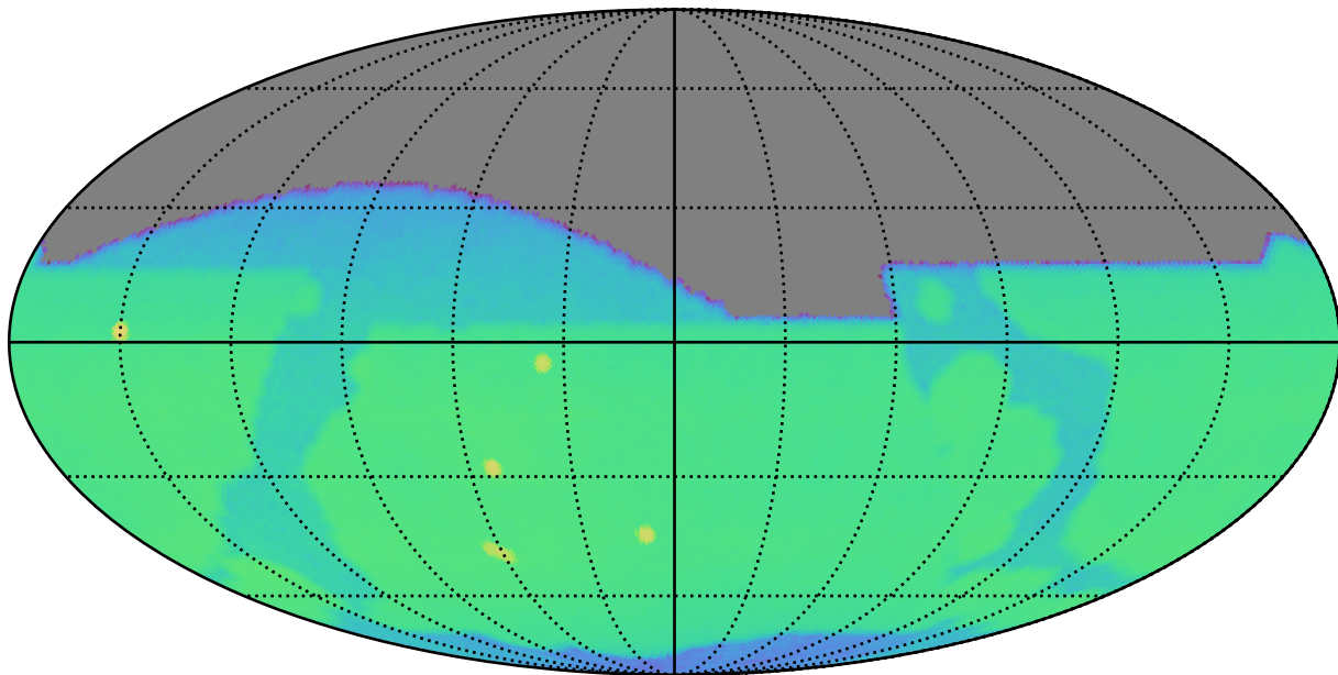
extra_ss_neo2_v3.4_10yrs r: CoaddM5
