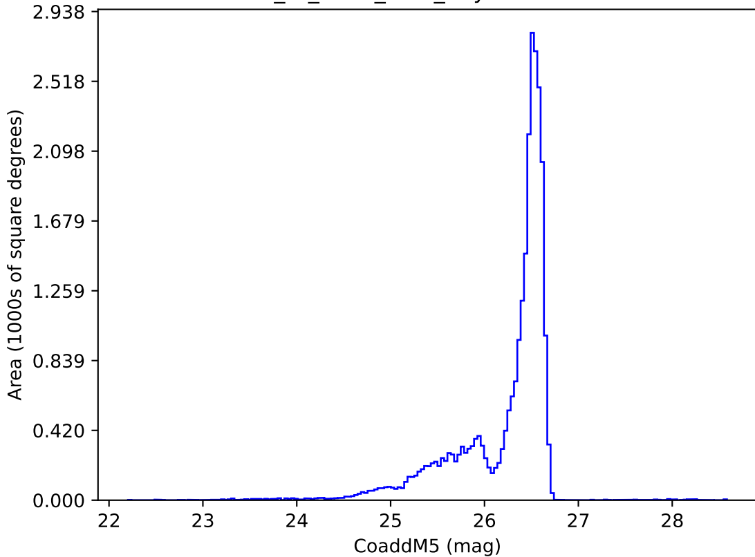
extra_ss_neo2_v3.4_10yrs i: CoaddM5
