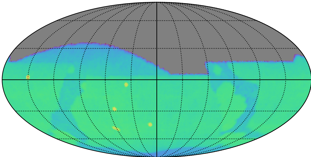
extra_ss_neo2_v3.4_10yrs g: CoaddM5
