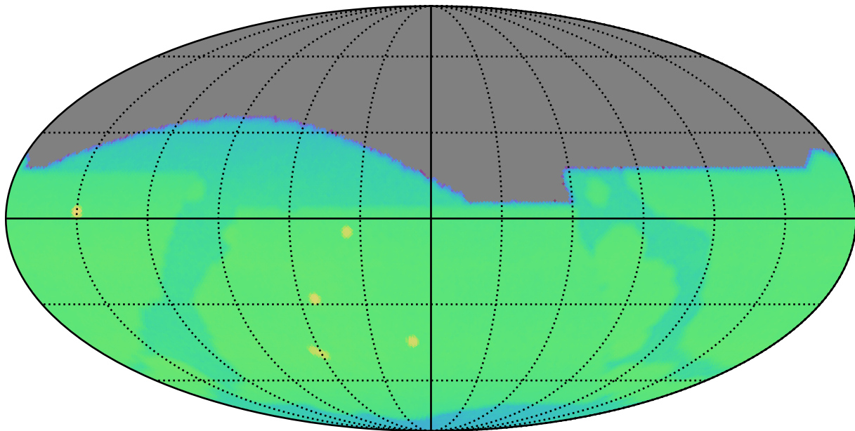
extra_ss_neo2_v3.4_10yrs : CoaddM5
