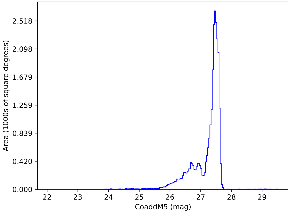
extra_ss_neo2_v3.4_10yrs : CoaddM5
