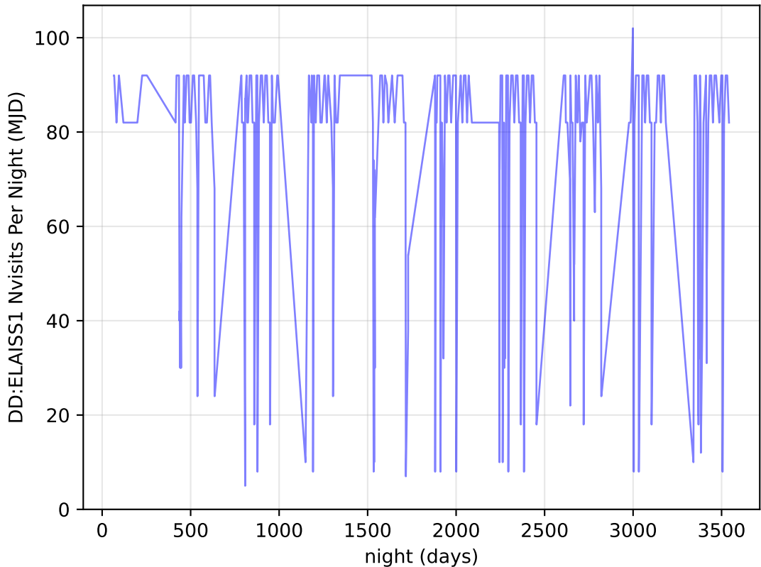
extra_ss_neo2_v3.4_10yrs all bands: DD:ELAISS1 Nvisits Per Night
