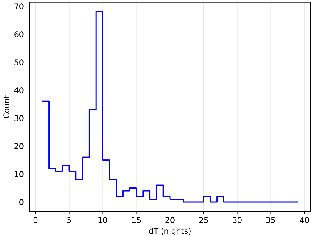
extra_ss_neo2_v3.4_10yrs all bands: DD:ELAISS1 Delta Nights Histogram
