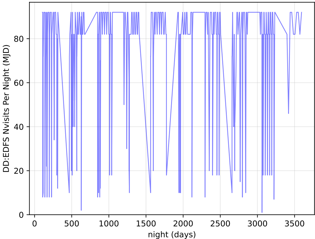
extra_ss_neo2_v3.4_10yrs all bands: DD:EDFS Nvisits Per Night
