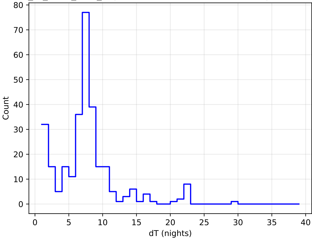
extra_ss_neo2_v3.4_10yrs all bands: DD:EDFS Delta Nights Histogram
